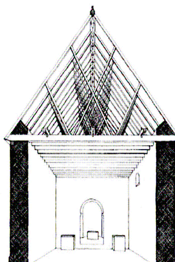
Principsektion i ett romanskt taklag, vilka ursprungligen har stått öppna mot kyrkorummet, ritning P. Sjömar, 1995.
